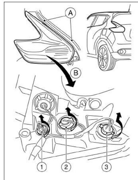
چراغ ترکیبی عقب
