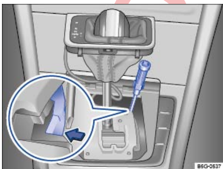
تصویر 154 باز کردن اضطراری قفل دسته دنده (نوع 1).
