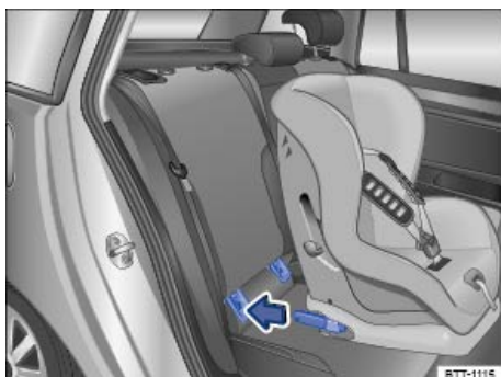
تصویر 28 طرح کلی: نصب صندلی ISOFIX با دسته‌های اتصال.
