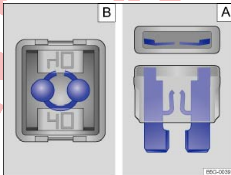
تصویر 285 فیوزهای سوخته: A فیوز تخت، B فیوز قالبی.
