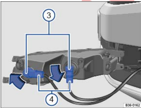
تصویر 277 لامپ چراغ جلو را عوض کنید.
