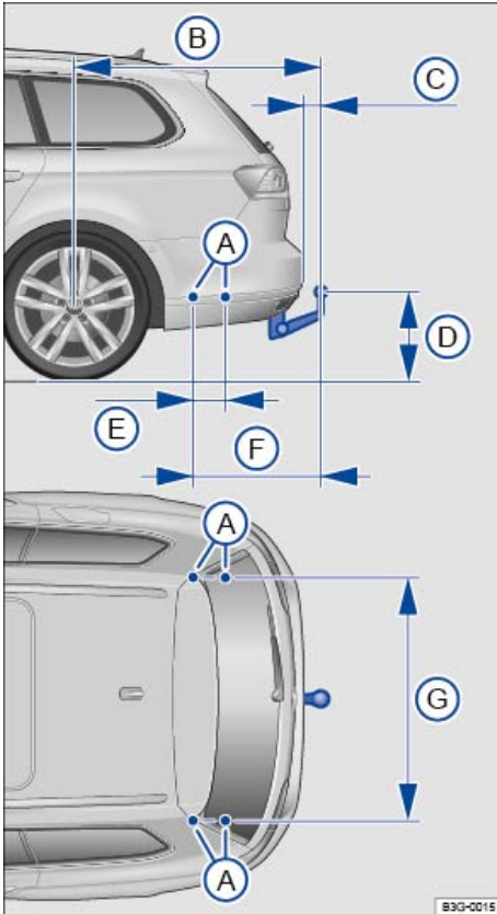
تصویر 265 ابعاد و نقاط اتصال برای نصب پایه یدک کش. (وارپانت).
