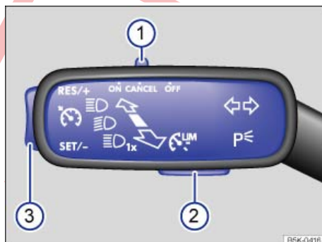
تصویر 161 در سمت چپ میله فرمان: کلیدها و دکمه‌هایی برای راه‌اندازی سیستم کروز کنترل (GRA).
