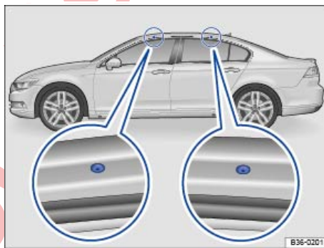
تصویر 260 زیر درزگیرهای درب جلو و عقب: نقاط اتصال پایه‌ها.
