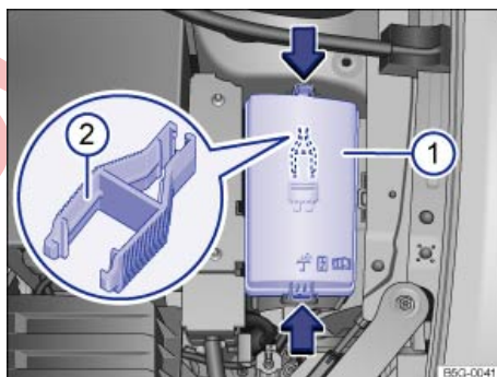
تصویر 282 درون محفظه موتور: پوشش 1 جعبه فیوز دارای انبرک پلاستیکی 2.
