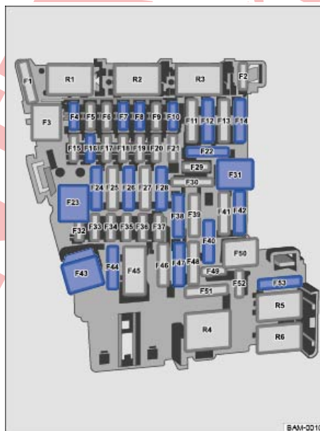
تصویر 283 در صفحه داشبورد: موقعیت فیوز.
