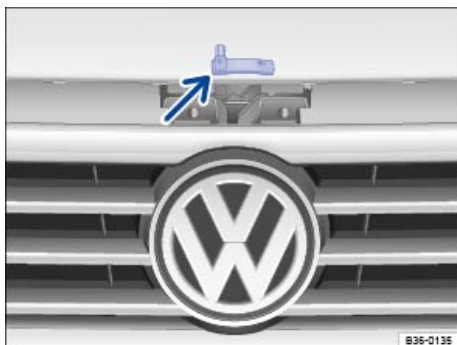
تصویر 296 بالای شبکه رادیاتور: اهرم نگه دارنده درب محفظه.
