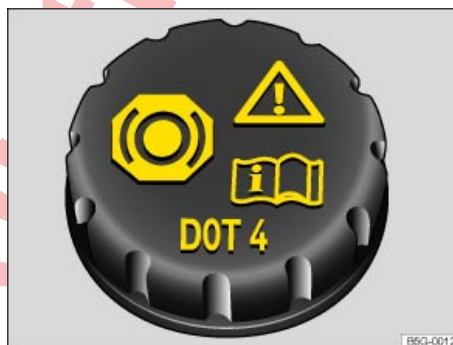
تصویر 303 در محفظه موتور: درب محفظه روغن ترمز.
