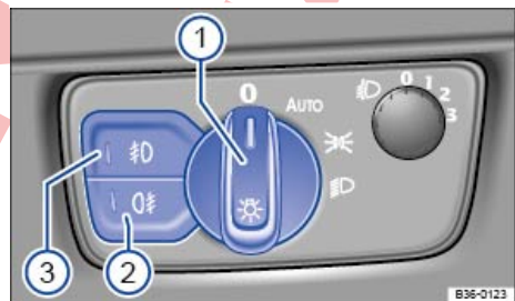
تصویر 117 کنار غریبک فرمان: کلیدهای نوری و دکمه ها برای چراغ های مشکن.
