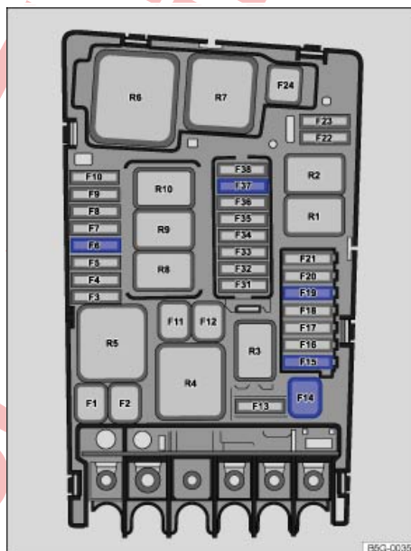
تصویر 284 در محفظه موتور: محل قرارگیری فیوز ها.
