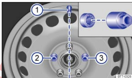
تصویر 319 تعویض چرخ: پیچ لاستیک ① و محل پیچ ضدسرفت ② یا ③.
