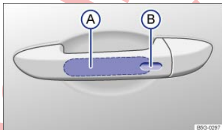
تصویر 79 سیستم روشن کردن و قفل کردن با دسترسی بدون کلید: سطح سنسور (A) برای باز کردن قسمت داخلی دستگیره درب و سطح سنسور (B) برای قفل کردن قسمت خارجی دستگیره درب.
