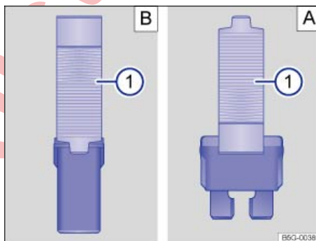
تصویر 286 فیوز را با انبرک پلاستیکی بیرون کشیده یا در جای خود قرار دهید: A فیوز تخت، B فیوز قالبی.
