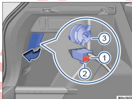
تصویر 243 جانی صندوق عقب: بیرون آوردن چراغ‌های عقب.
