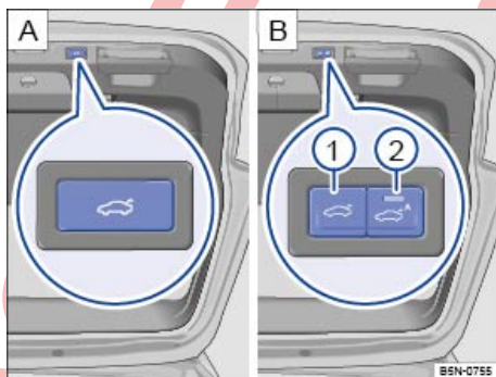
تصویر 83 داخل صندوق عقب: دکمه برای بستن برقی درب صندوق عقب.
