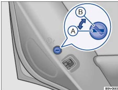
تصویر 73 در درب عقب سمت چپ: قفل کودک (A) غیرفعال، (B) فعال.
