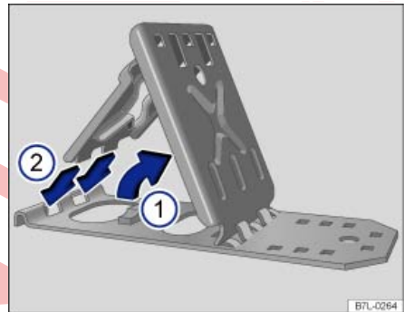
تصویر 236 باز کردن نگهدارنده تاشوی چرخ.
