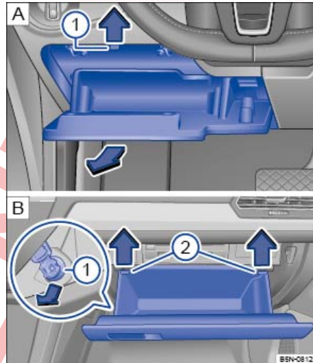
تصویر 244 در سمت راننده داخل صفحه داشبورد؛ پوشش جعبه فیوز.
