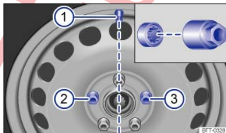
تصویر 281 تعویض چرخ: پیچ لاستیک ۱ و محل پیچ ضدسرقت ۲ یا ۳.
