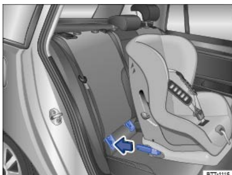
تصویر 27 طرح کلی: نصب صندلی ISOFIX با دسته‌های اتصال.
