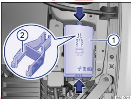
تصویر 246 درون محفظه موتور: پوشش ① جعبه فیوز دارای انبرک پلاستیکی ②.
