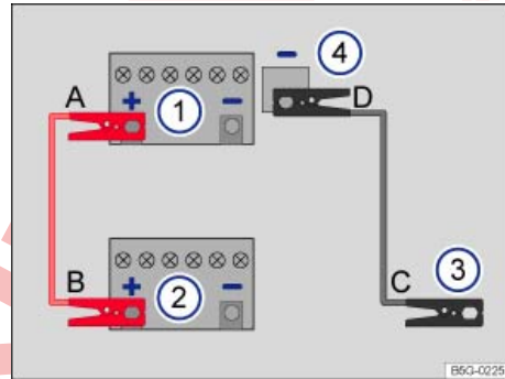
تصویر 253 نقشه نحوه اتصال کابل‌های شارژ (باتری خودرو داخل محفظه موتور).
