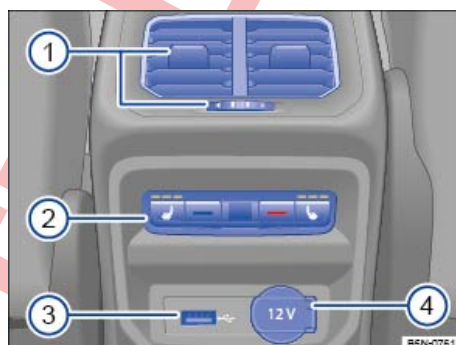
تصویر 46 نمای کلی بخش عقب کنسول وسط.
