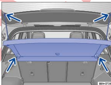
تصویر 216 در صندوق عقب: ول کردن و جدا کردن درپوش صندوق عقب.
