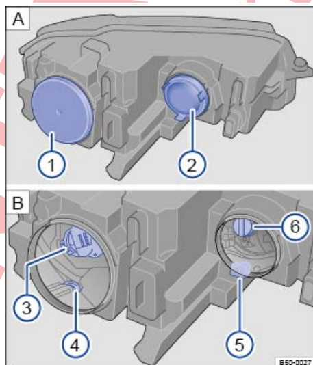
تصویر 240 درون محفظه موتور: پوشش‌ها و B لامپ‌ها در سمت چپ چراغ‌های جلو.
