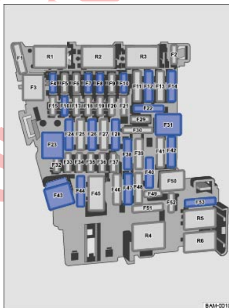
تصویر 247 در صفحه داشبورد: موقعیت فیوز.
