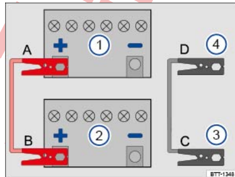
تصویر 254 نقشه نحوه اتصال کابل‌های شارژ (باتری خودرو در صندوق عقب).
