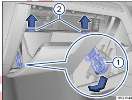
تصویر 245 پوشش جعبه فیوز در صفحه داشبورد؛ در خودروهای با فرمان سمت راست سمت سر نشین جلو.
